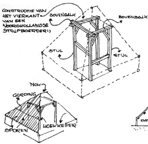
Constructie van een stolpboerderij.
