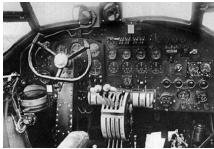
Overzicht van het instrumentenpaneel van de piloot van een Lancaster. Bron: www.strijdbewijs.nl
